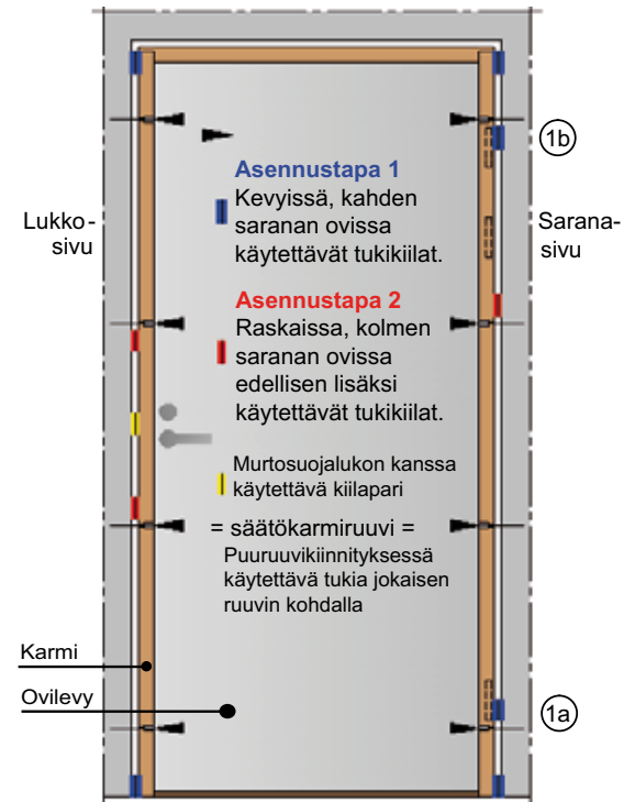
Kuva 1 Karmin kiinnittämien oviaukkokoon
